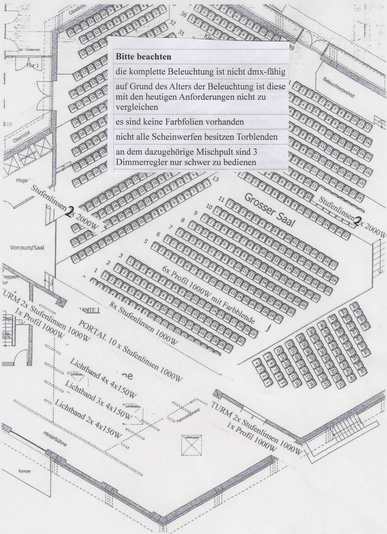
Vorhandene Beleuchtung Verdo Hitzacker
